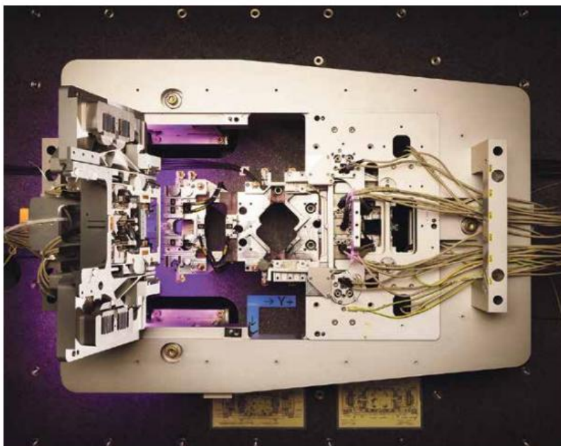
"Reticle stage", onderdeel van een chipmachine van ASML.
